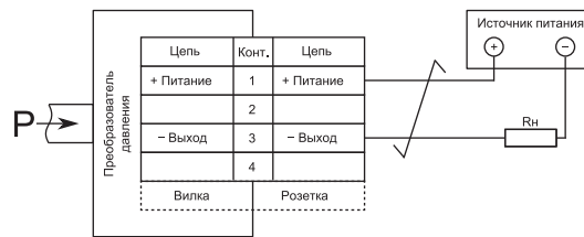
Схема подключения преобразователей общепромышленного исполнения
