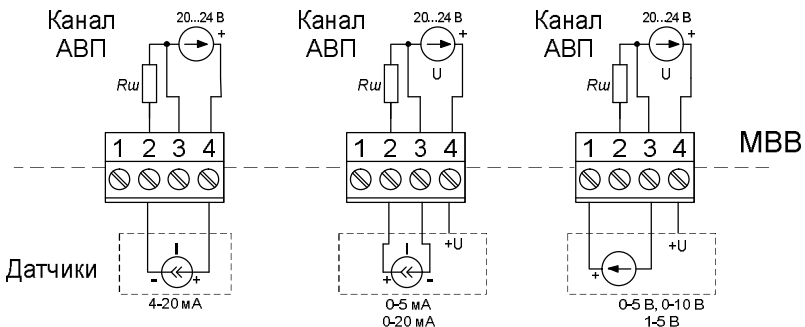
Рисунок 1.4 Варианты подключения датчиков к каналам АВП
